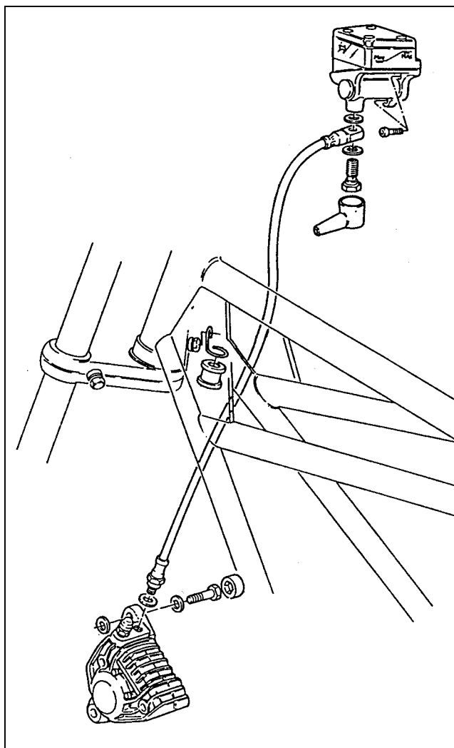
SYSTÈME AVANT DROIT (FIG. 335)
